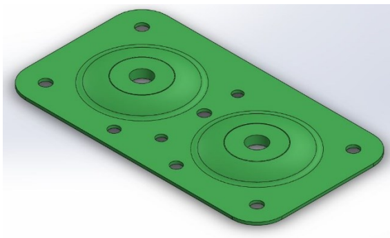
DIAFRAGMA PULSADOR BOUMATIC GASCOIGNE MELOTTE (Cód. 0196)
